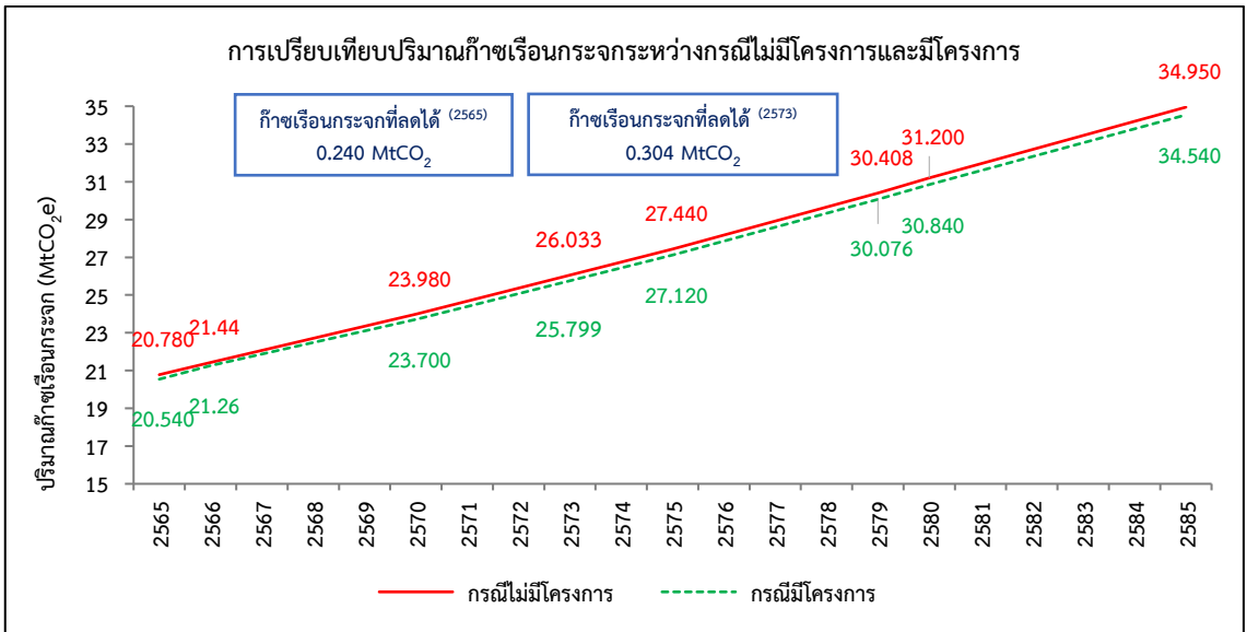
รูปที่ 2.6.2-31 การเปรียบเทียบปริมาณก๊าซเรือนกระจกระหว่างกรณีไม่มีโครงการและกรณีมีโครงการ ของโครงการรถไฟฟ้าคู่ ระยะที่ 1 รวม 7 เส้นทาง
