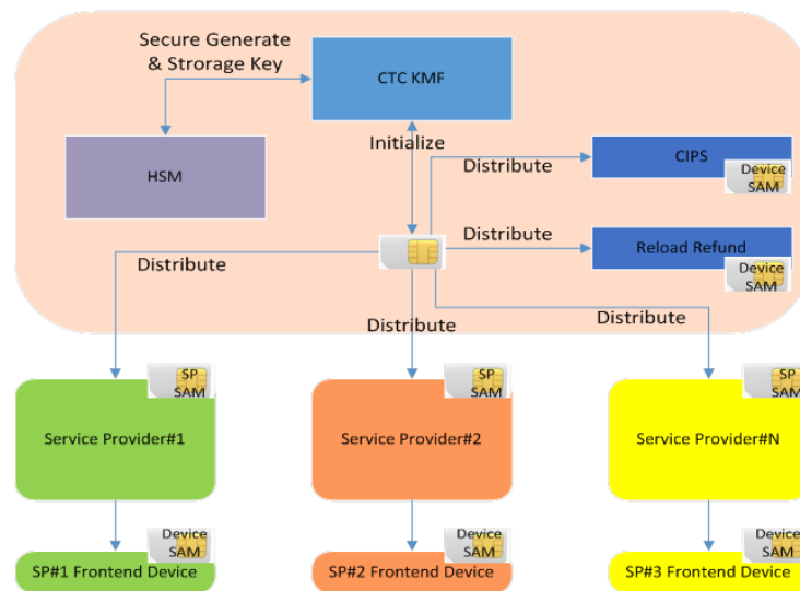
แผนภูมิที่ 3-27 ภาพรวมระบบจัดการความปลอดภัย
