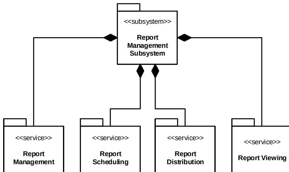
แผนภูมิที่ 3-11 ภาพรวม Report Management Subsystems
