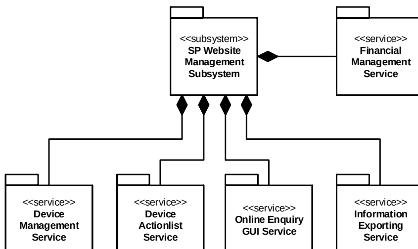
แผนภูมิที่ 3-21 ภาพรวม SP Website Subsystems
