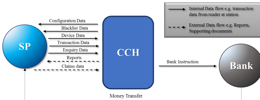
แผนภูมิที่ 3-28 การเชื่อมต่อระหว่างหน่วยงานที่เกี่ยวข้อง
