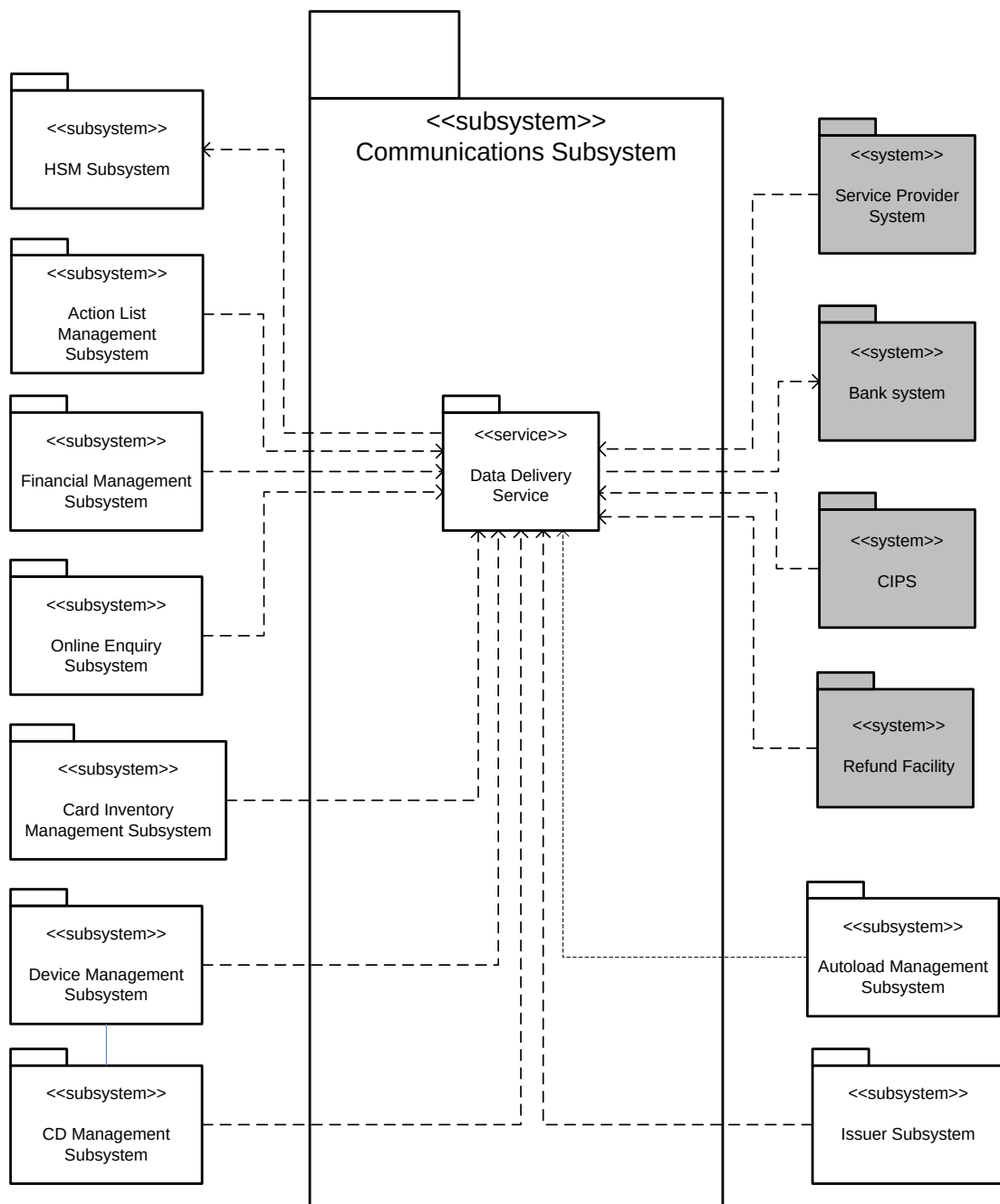
แผนภูมิที่ 3-17 ภาพรวม Communication Management Subsystems
