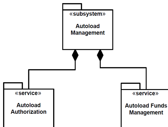
แผนภูมิที่ 3-13 ภาพรวม Autoload Management Subsystems
