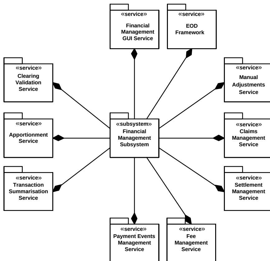
แผนภูมิที่ 3-7 ภาพรวม Financial Management Subsystems
