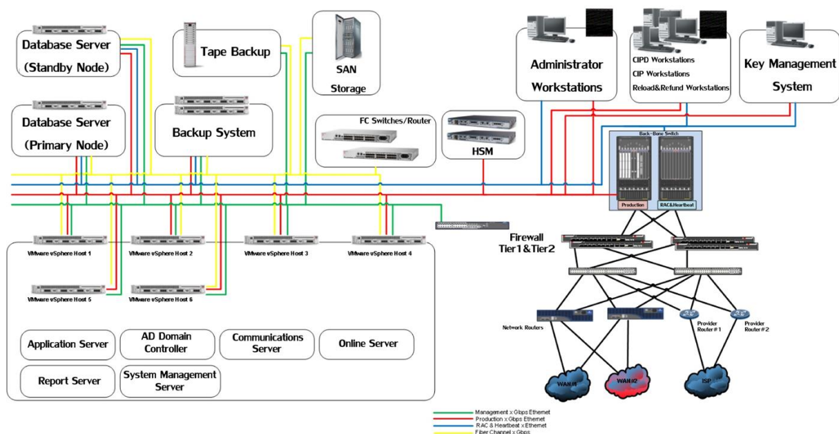
แผนภูมิที่ 3-23 สถาปัตยกรรมเครือข่าย
