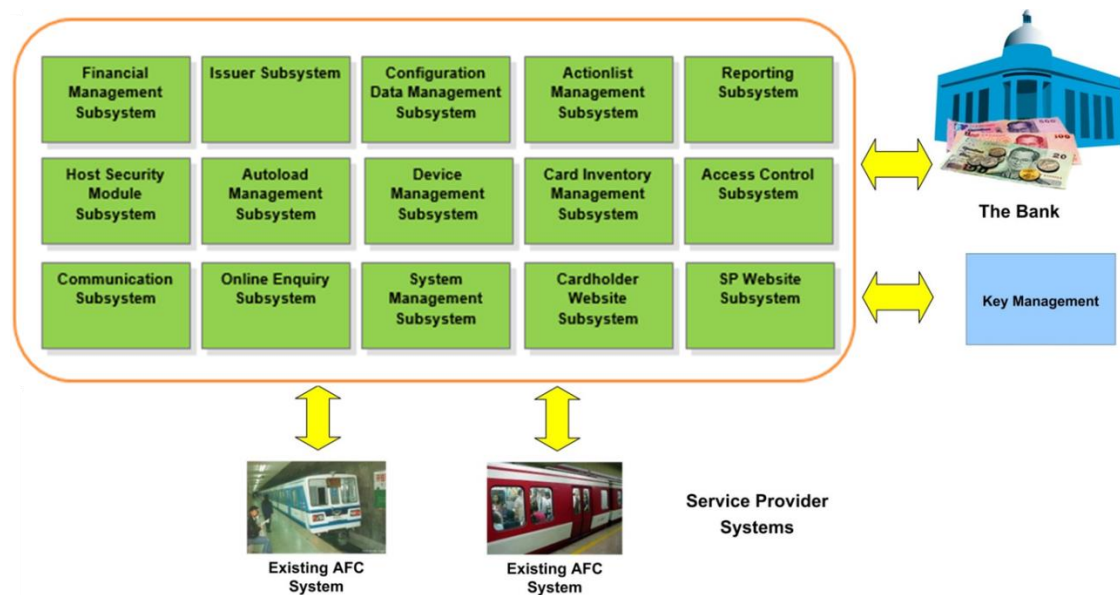
แผนภูมิที่ 3-6 สถาปัตยกรรมระบบ
