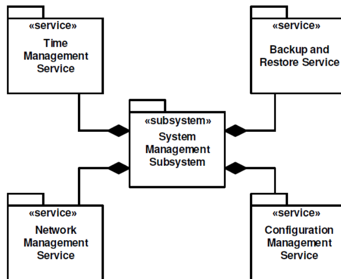
แผนภูมิที่ 3-20 ภาพรวม System Management Subsystem
