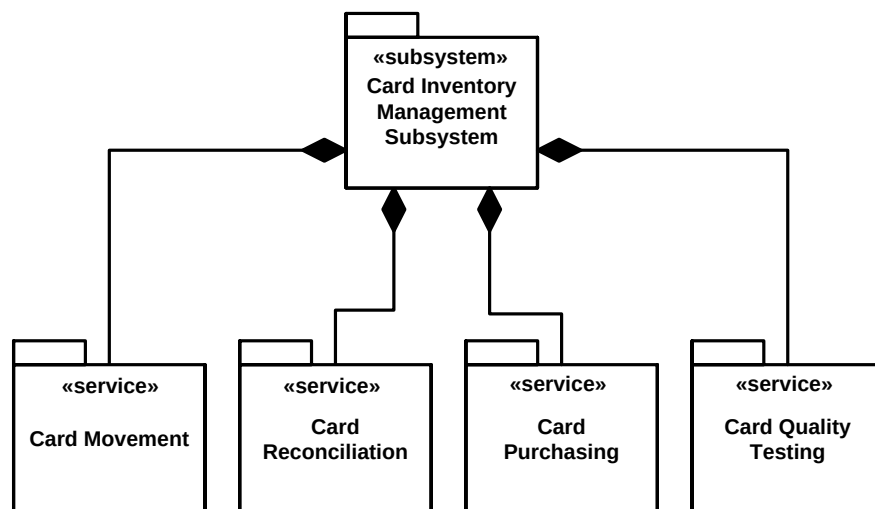
แผนภูมิที่ 3-15 ภาพรวม Card Inventory Subsystems
