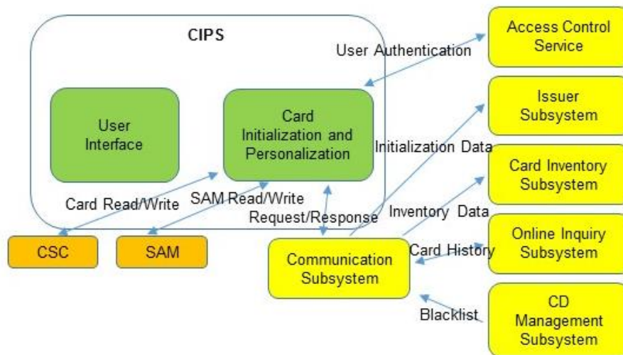
แผนภูมิที่ 3-25 เครื่องจัดการข้อมูลบัตรและข้อมูลบัตรส่วนบุคคล
