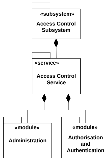
แผนภูมิที่ 3-18 ภาพรวม Access Control Subsystem
