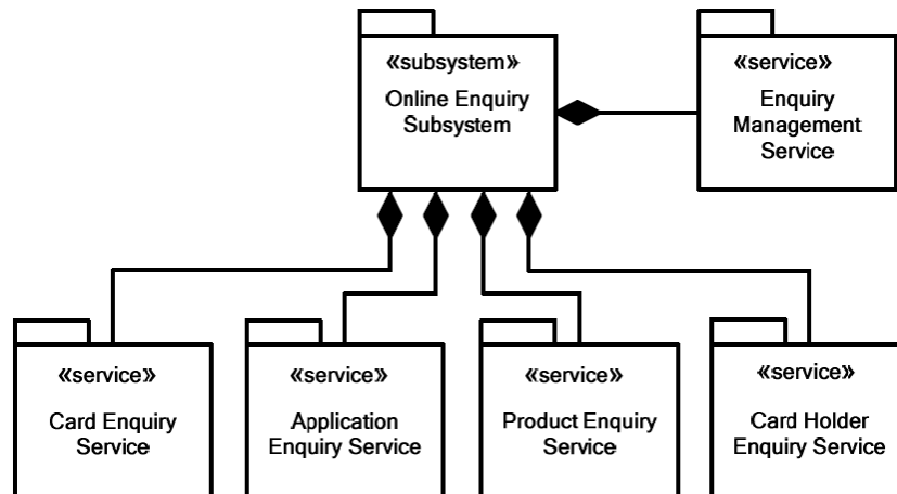
แผนภูมิที่ 3-19 ภาพรวม Online Enquiry Subsystem
