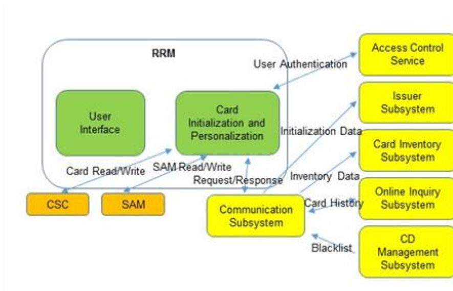
แผนภูมิที่ 3-26 เครื่องเติมเงิน/คืนเงินกับการติดต่อกับส่วนต่างๆ
