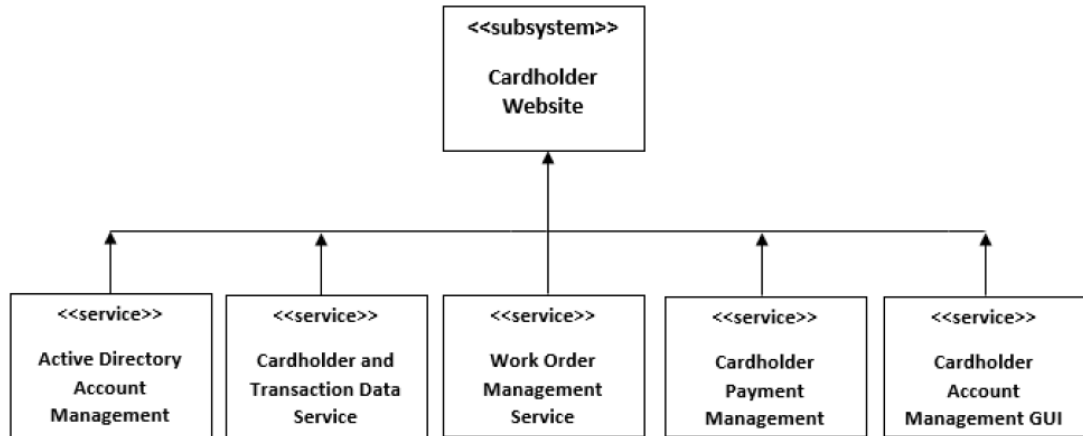
แผนภูมิที่ 3-16 ภาพรวม Cardholder Website Subsystems
