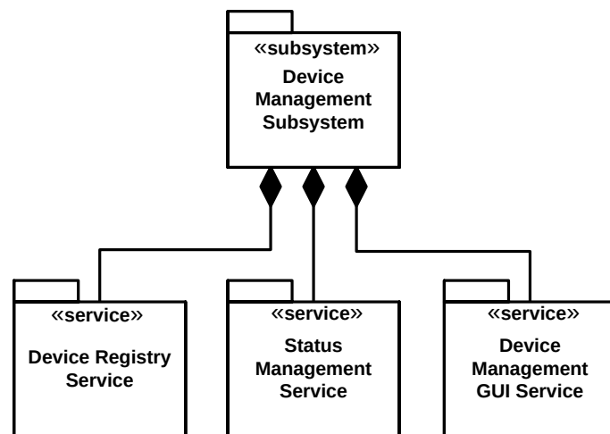
แผนภูมิที่ 3-14 ภาพรวม Device Management Subsystems
