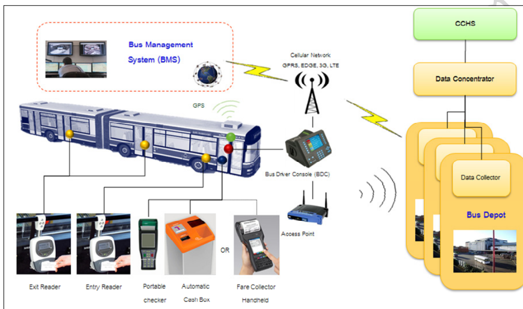
แผนภูมิที่ 5.3-4 ระบบการจัดเก็บรายได้ในส่วน รถโดยสารประจำทาง
