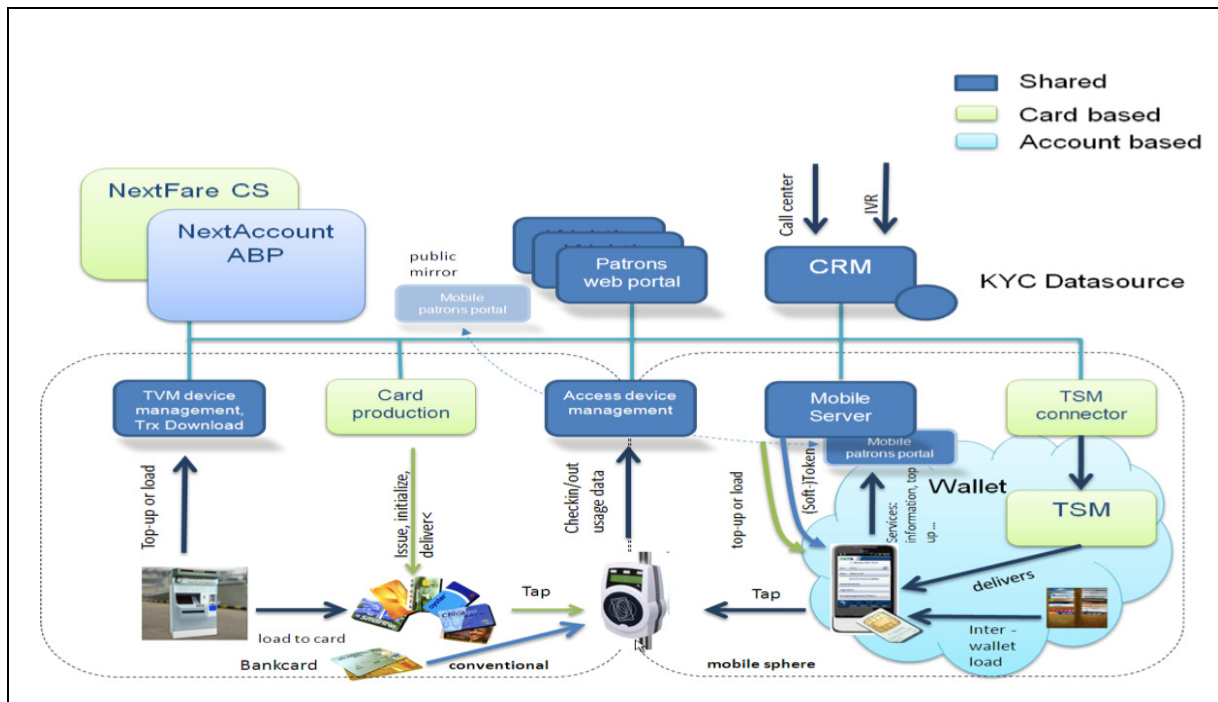
แผนภูมิที่ 3.2-6 ตัวอย่างการใช้งาน Account Based System ในลอนดอน
