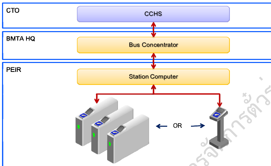
แผนภูมิที่ 5.3-6 การเชื่อมต่อระบบเรือโดยสาร
