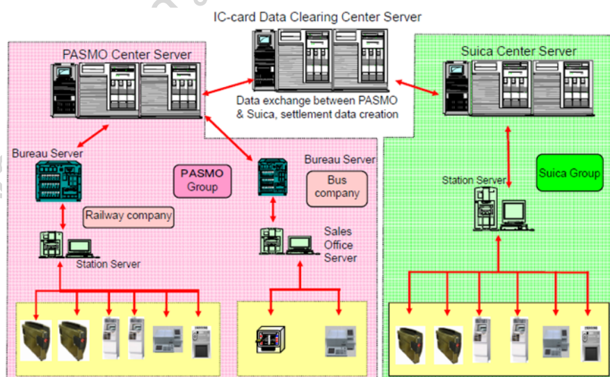
แผนภูมิที่ 2.3-27 การเชื่อมต่อกันระหว่างระบบบัตร SUICA และ PASMO
