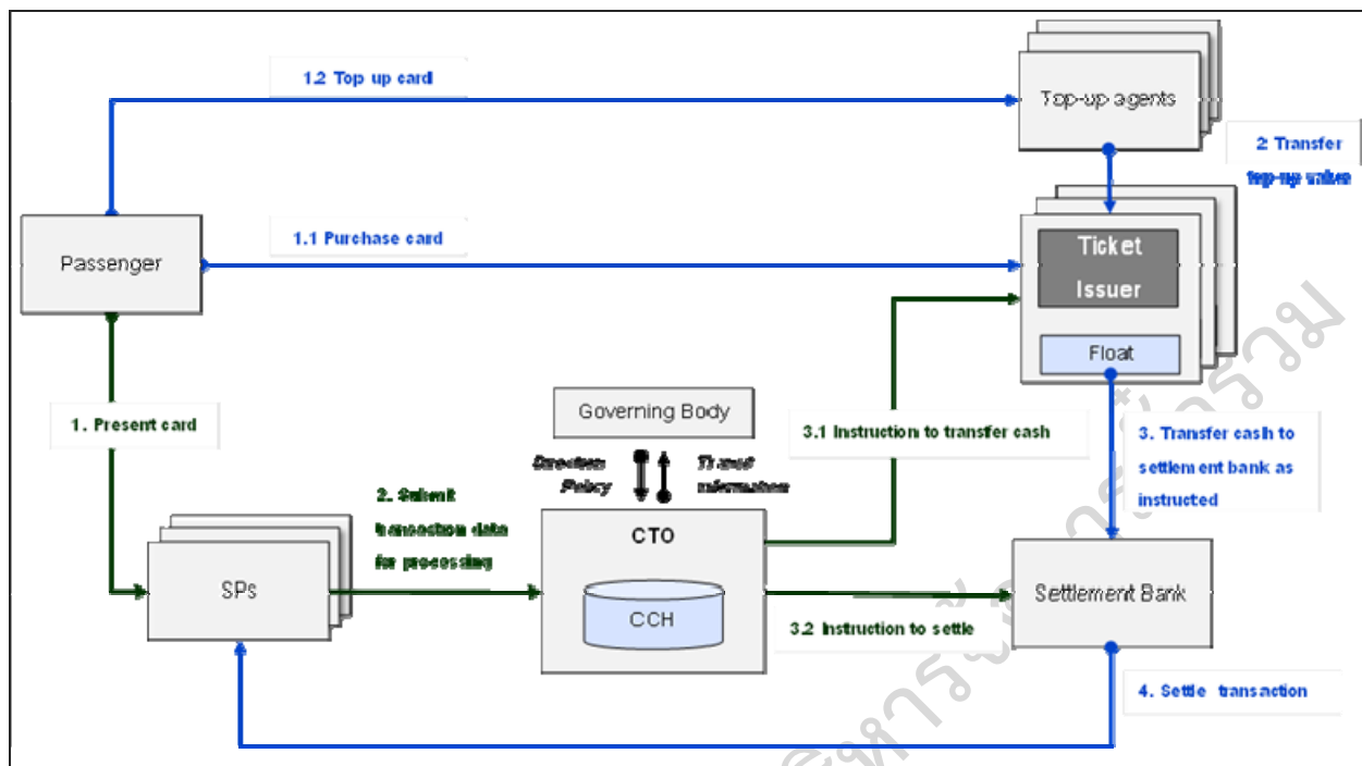
แผนภูมิที่ 4.4-1 ภาพรวมการดำเนินงานของระบบตั๋วร่วม
