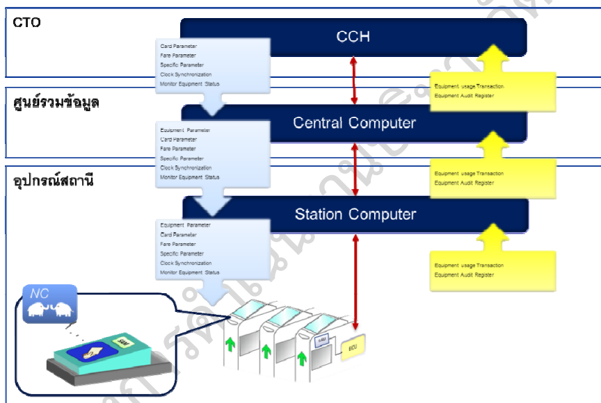
แผนภูมิที่ 5.3-3 การปรับปรุงอุปกรณ์ระบบรถไฟฟ้า
