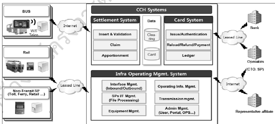
แผนภูมิที่ 4.4-2 ตัวอย่างโครงสร้างระบบของศูนย์บริหารจัดการรายได้กลาง
