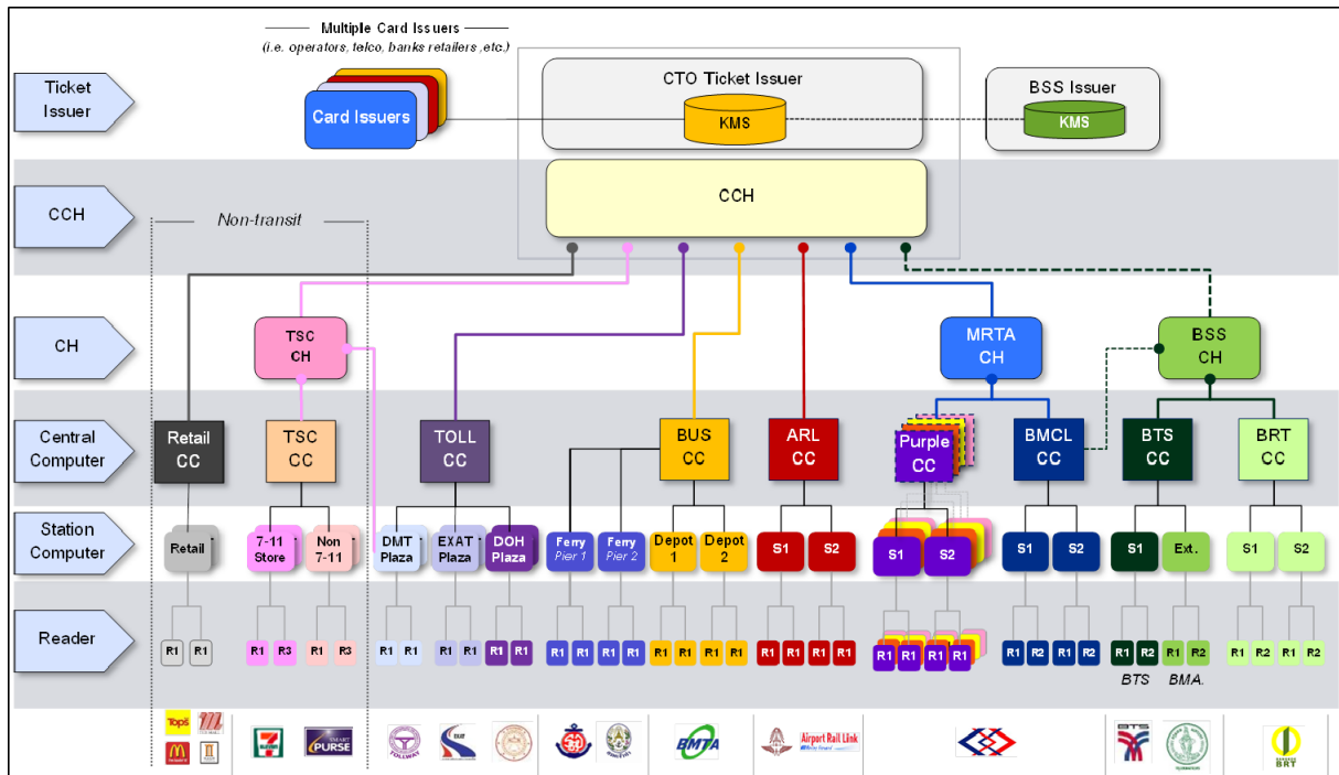
แผนภูมิที่ 5.3-2 รูปแบบโครงสร้างระบบตัวร่วม รูปแบบที่ 2
