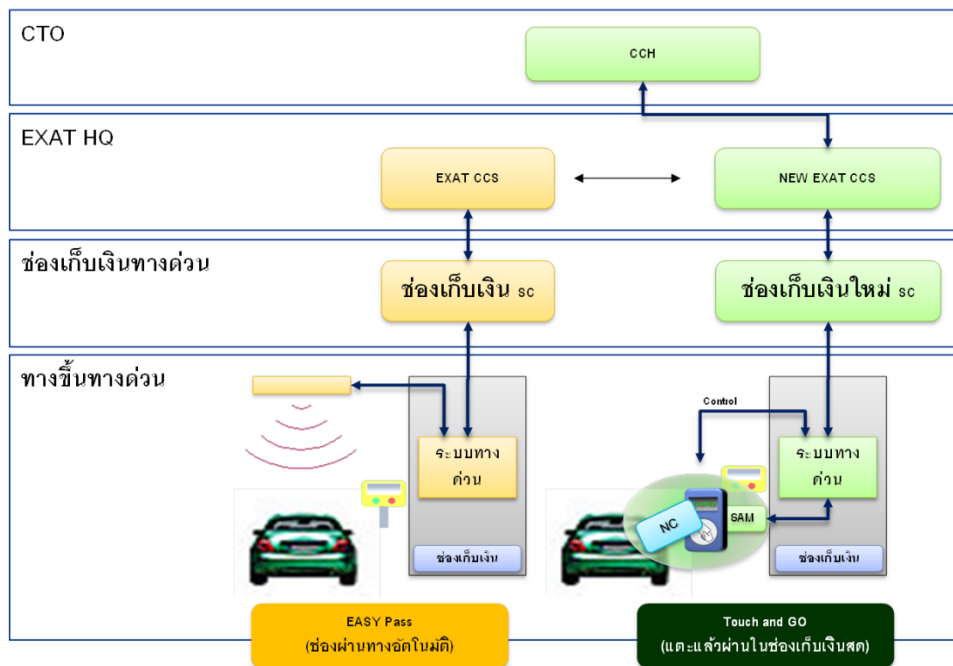
แผนภูมิที่ 5.3-5 ระบบการจัดเก็บรายได้แบบ Touch &amp; Go
