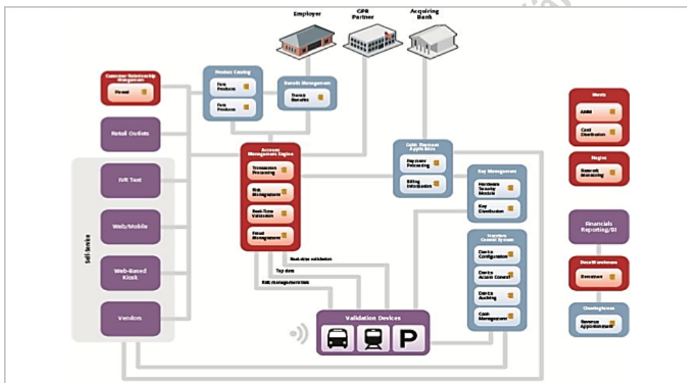
แผนภูมิที่ 2.3-38 Open Payment AFC System in London
